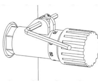
Рис. 2 Схема установки терморегулятора.
